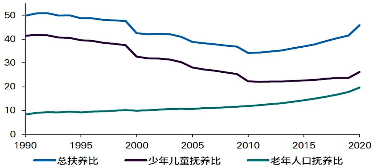
图7 人口抚养比，%
